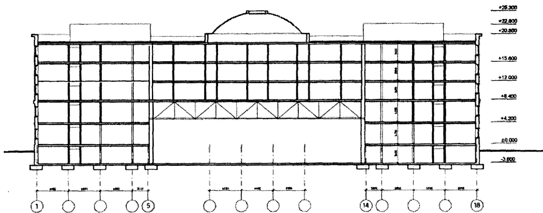
Рисунок Н.3 - Продольный разрез
