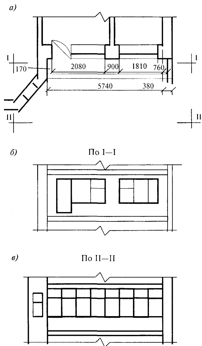
Рисунок Т.1 - План (а), разрез (б) по сечению I-I плана и фасад (в) по сечению II-II остекленного балкона многоэтажного жилого здания
