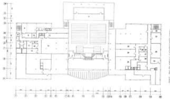
Рисунок Н.2 - План цокольного этажа
