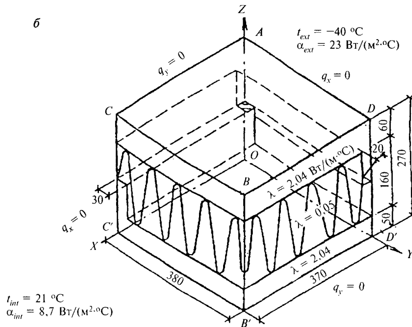
Рисунок К.2 - Конструкция панели совмещенной крыши ( a ) и схема расчета конструкции панели совмещенной крыши ( б )
