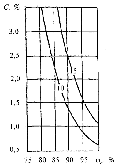
Рисунок III.2 - Изолинии сорбционного влагосодержания керамзитобетона \rho_0 = 1200 кг/м 3 , содержащего хлорид калия, при изменении относительной влажности воздуха \varphi_a , %, и массового солесодержания C , %
