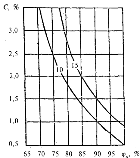
Рисунок III.1 - Изолинии сорбционного влагосодержания керамзитобетона \rho_0 = 1200 кг/м 3 , содержащего хлорид натрия, при изменении относительной влажности воздуха \varphi_a , %, и массового солесодержания C , %
