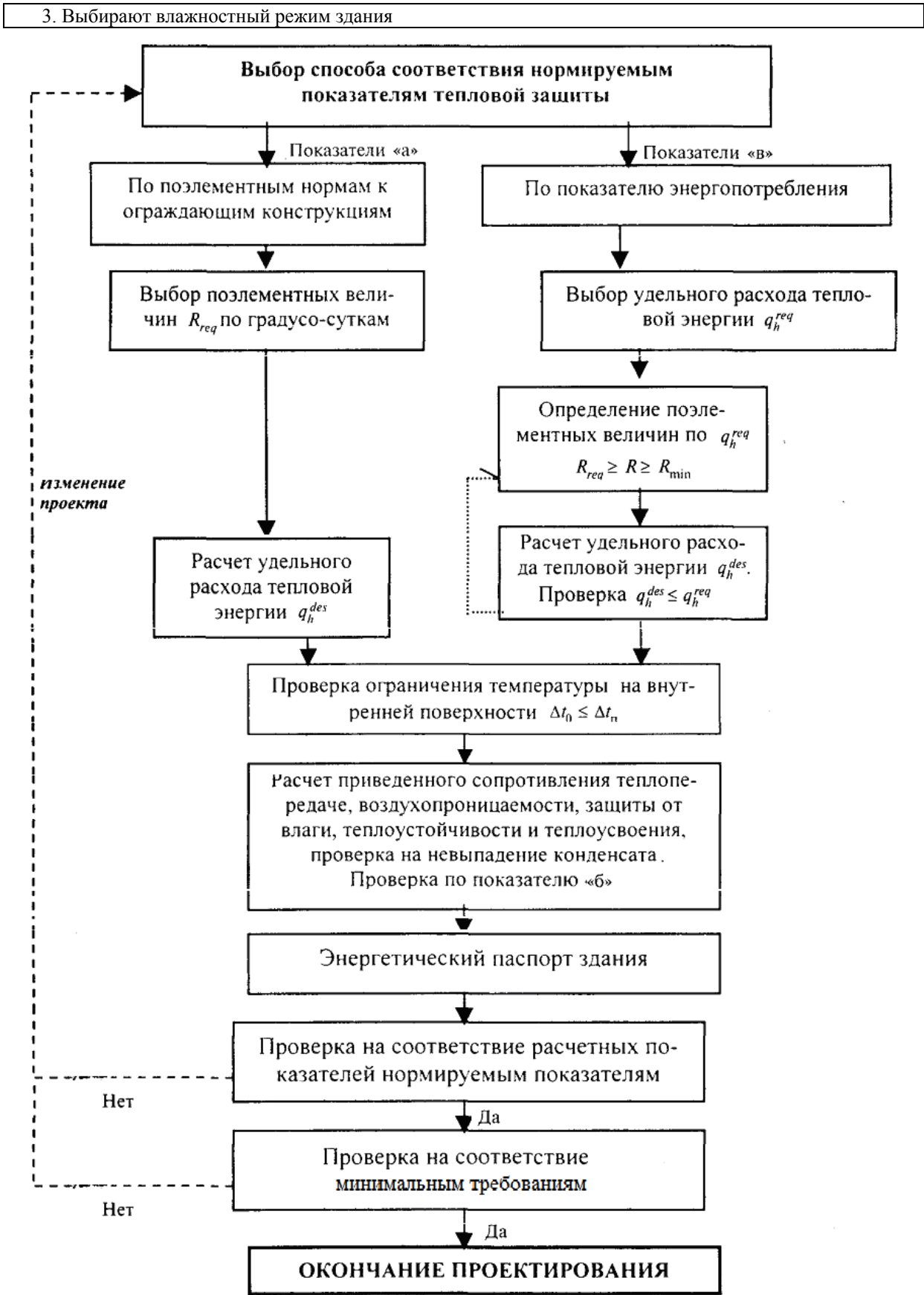
Рисунок 1 - Схема проектирования тепловой защиты зданий
