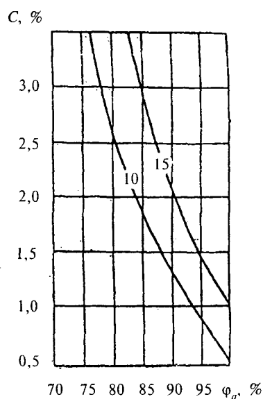
Рисунок Ш.6 - Изолинии сорбционного влагосодержания керамзитобетона \rho_0 = 1200 кг/м 3 , содержащего NaCl - 30 %, KCl - 60 %, MgCl 2 - 10 %, при изменении относительной влажности воздуха \phi_a , %, и массового солесодержания C , %, в стенах цехов сушки
