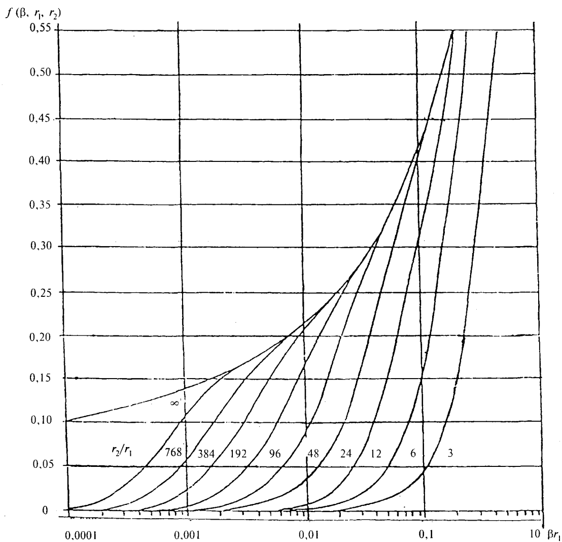
Рисунок M.1 - Функция f(\beta, r_1, r_2)
