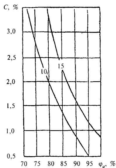
Рисунок III.4 - Изолинии сорбционного влагосодержания керамзитобетона \rho_0 = 1200 \text{кг/м}^3 , содержащего NaCl - 60 %, KCl - 30 %, \text{MgCl}_2 - 10 %, при изменении относительной влажности воздуха \varphi_a , %, и массового солесодержания C , %, в стенах флотофабрик
