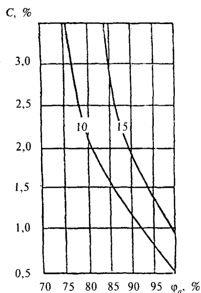
Рисунок Ш.5 - Изолинии сорбционного влагосодержания керамзитобетона \rho_0 = 1200 кг/м 3 , содержащего NaCl - 50 %, KCl - 30 %, MgCl 2 - 10 %, при изменении относительной влажности воздуха \phi_a , %, и массового солесодержания C , %, в стенах цехов дробления руды
